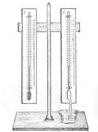
Рисунок 6 – Психрометр
