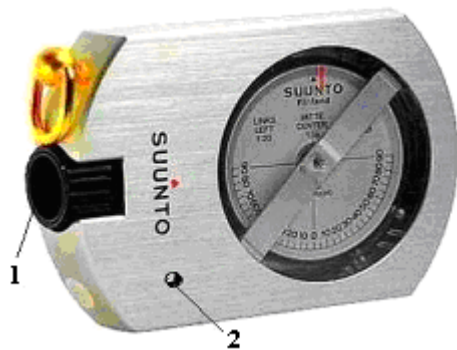
1 – окуляр; 2 – дальномер
