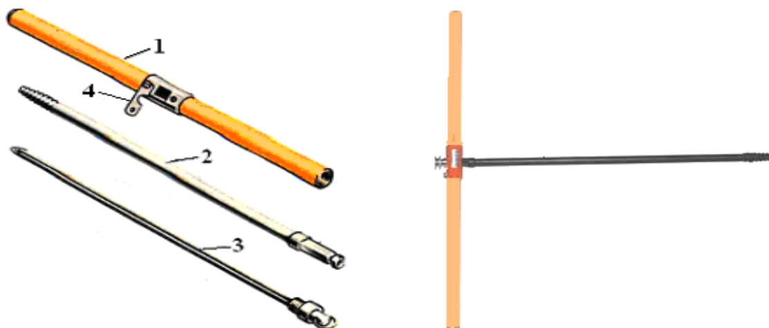
1 – футляр-рукоятка; 2 – бур; 3 – щуп; 4 – фиксатор
