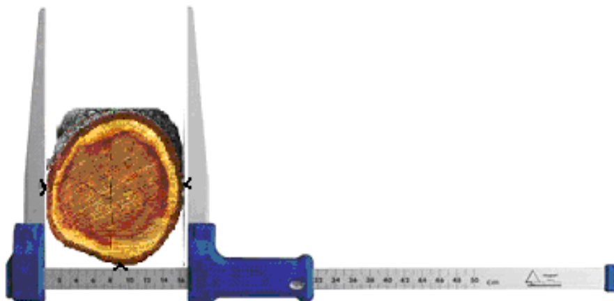
Рис. 1.2. Мерная вилка
