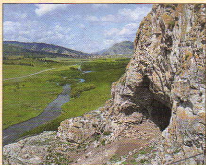
Вход в Усть-Канскую пещеру, палеолитическую стоянку. Алтай
