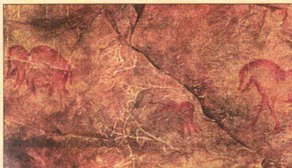
Капова пещера на Южном Урале. Изображения мамонтов, лошадей и носорога
